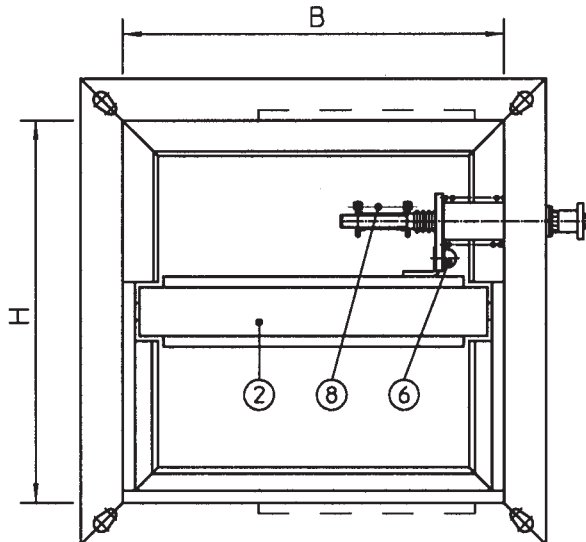
Ansicht A
